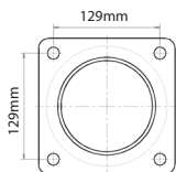
vloerplaat SOLARIS
