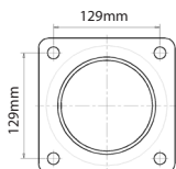
Baseplate SOLARIS
